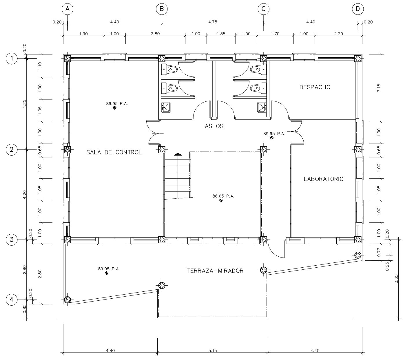
PLANTA PRIMERA ESCALA 1:50
