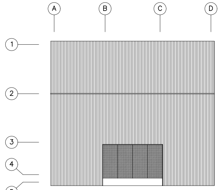
PLANTA DE CUBIERTA ESCALA 1:100
